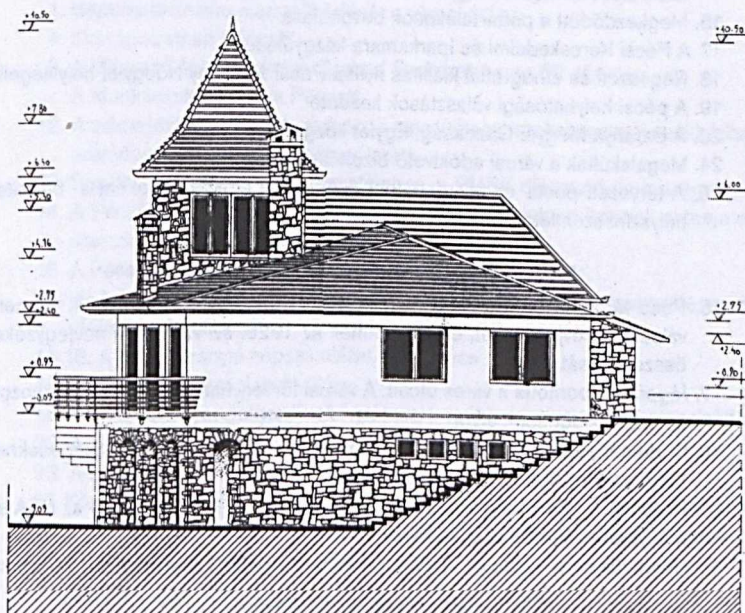
DÉLI HOMLOKZAT M=1:100
