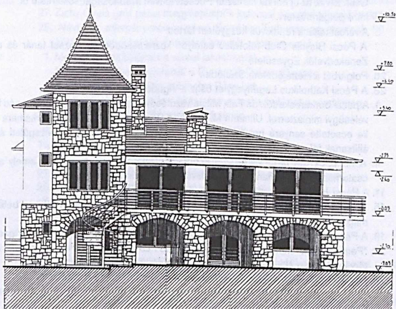
NYUGATI HOMLOKZAT M=1:100
