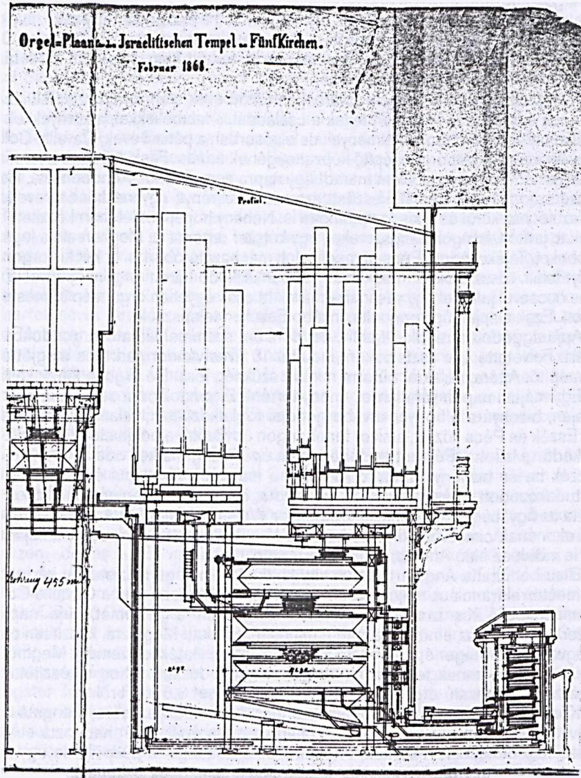
Az orgona műszaki-szerelési terve. Hosszmetszet
