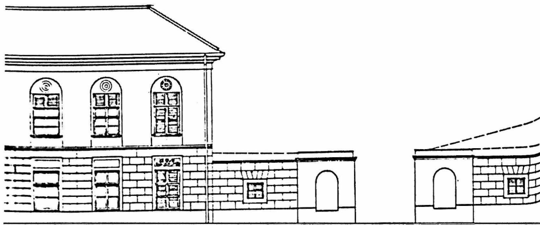
A főhomlokzat nézetrajza
