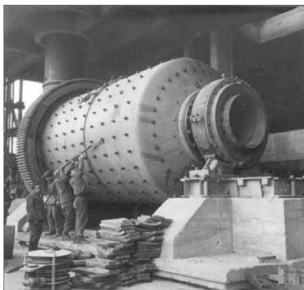
A 4,5 m hosszú, 3 m átmérőjű szénőrlő malom szerelése
