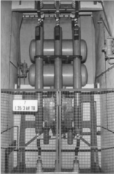
A 35 kilovoltos alállomás kapcsolója
