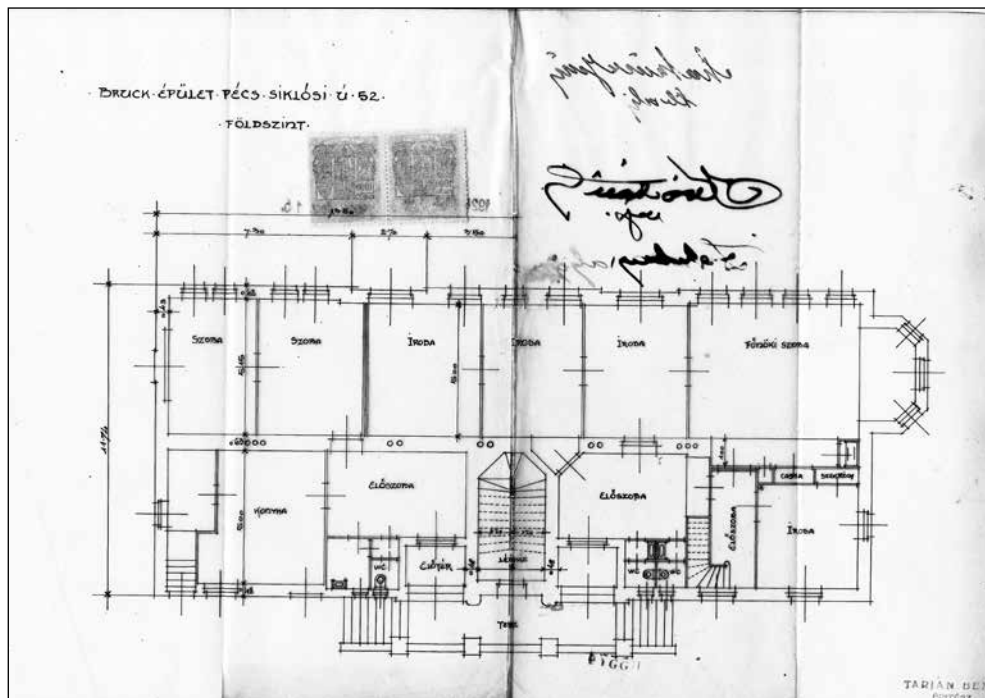
Siklósi utca 52. A földszint tervváltozata. Tarján Benő, 1923.
