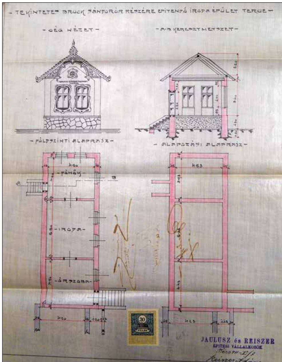
Siklósi utca 52. Bruck Sándor telkén az első faraktár és irodaépület tervrajza. Reisner Ádám és Jaulusz Gyula, 1911.
