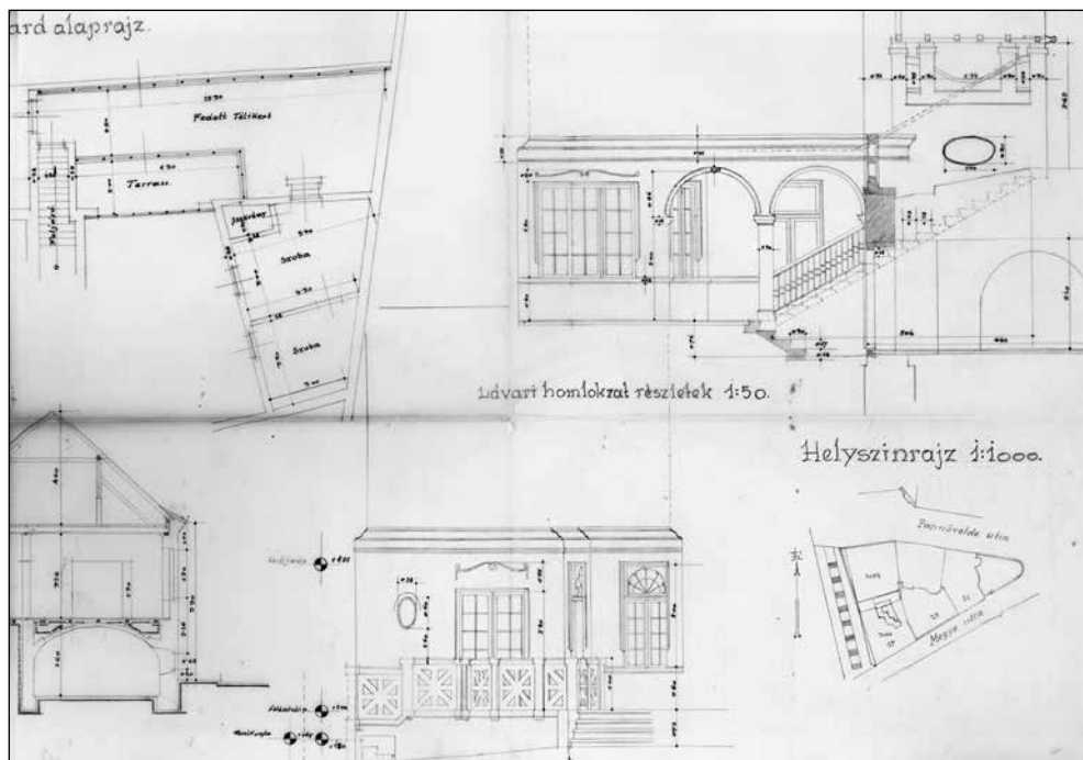
Bruck Sándor házának átalakítása. Udvari homlokzatterv. Tarján Benő, 1922.
