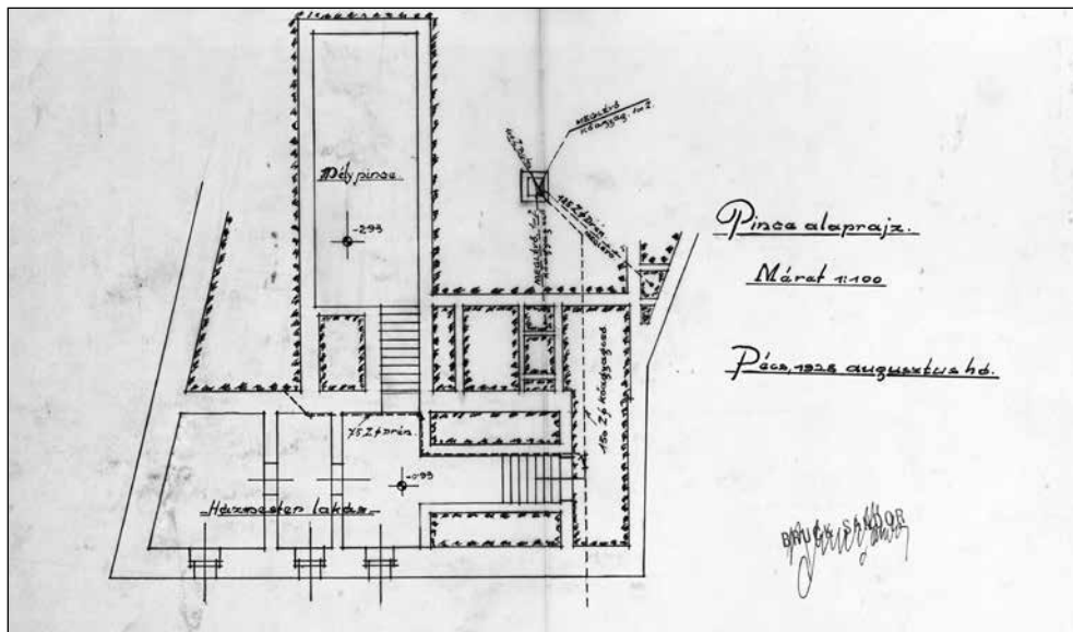
Bruck Sándor házának átalakítása. A házmesterlakás és a mélypince tervrajza. Tarján Benő, 1928.
