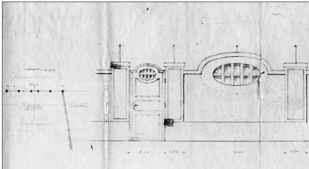
Bruck Sándor házának átalakítása. Kerítésterv a Papnövelde utcában. Tarján Benő, 1927.
