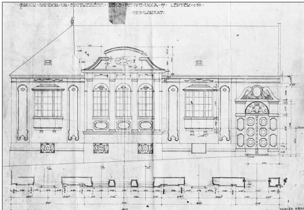
Bruck Sándor házának átalakítása. Homlokzatterv. Tarján Benő, 1922.
