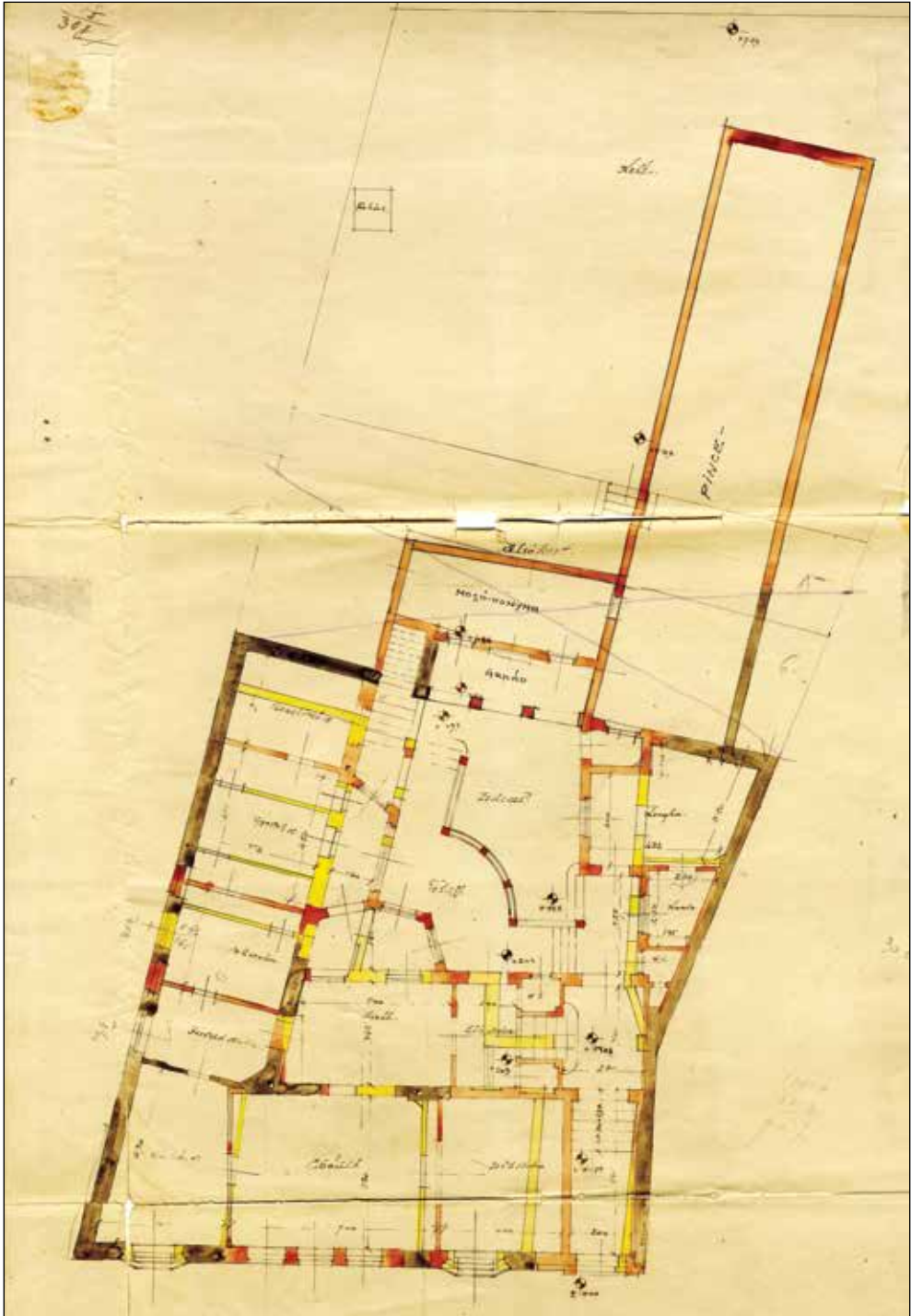
Bruck Sándor házának átalakítása. Alaprajz. Tarján Benő, 1922.
